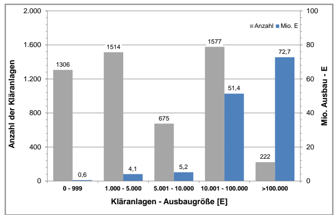
Abbildung 1: Anzahl und Ausbaugrößen der am DWA-Leistungsnachweis 2022 beteiligten Kläranlagen nach Größenklassen
