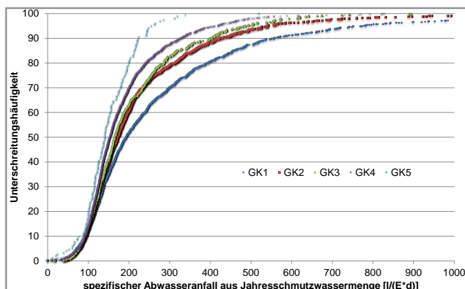
Abbildung 5: Summenhäufigkeit der spezifischen Jahresabwasser- und Jahresschmutzwassermengen nach Größenklassen
