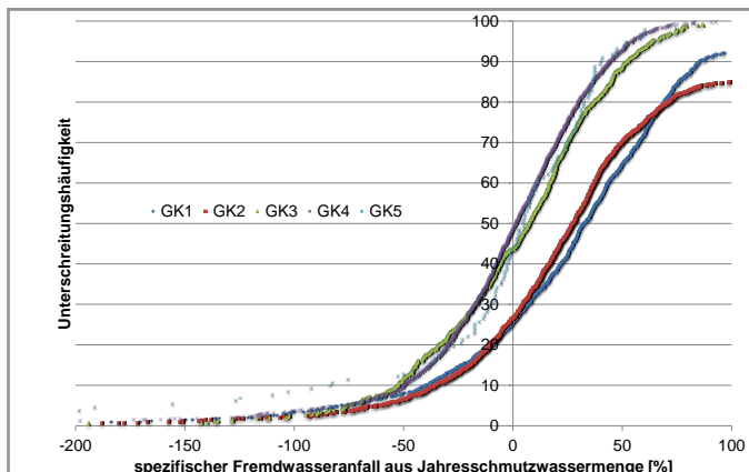
Abbildung 6: Summenhäufigkeit der spezifischen Fremdwassermengen und -anteile aus den JSM nach Größenklassen
