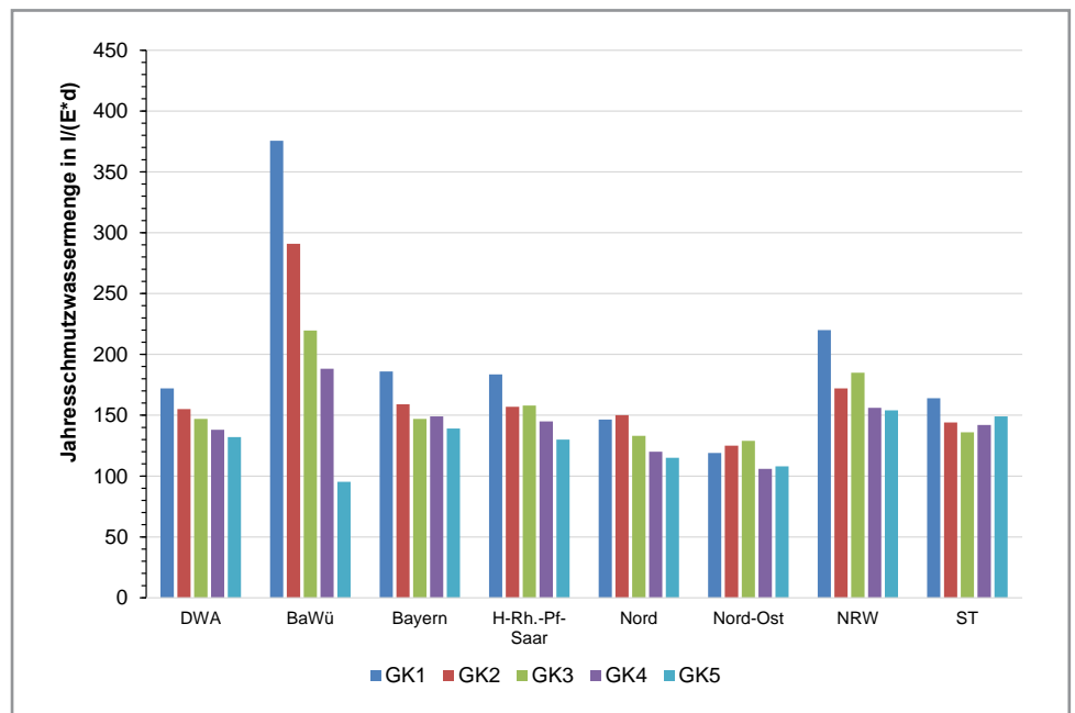
Abbildung 3: spezifische Zuflüsse nach Größenklassen und DWA-Landesverbänden (Medianwerte)
