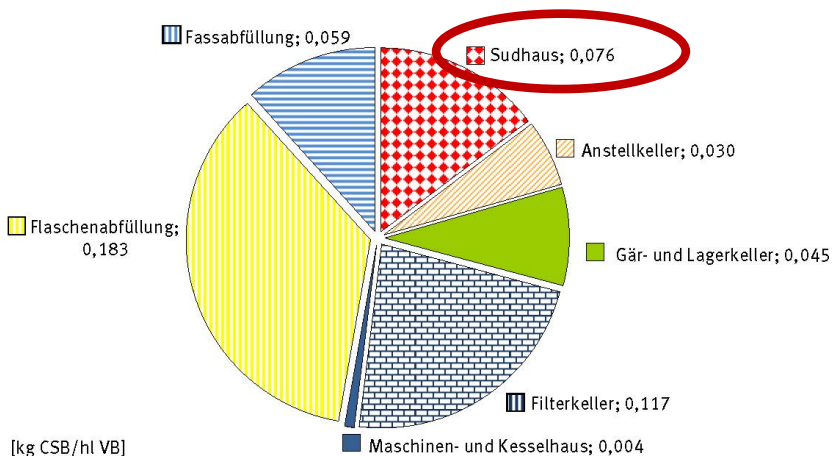
Bild 3: Spezifische CSB-Frachten aus den Abteilungen einer Großbrauerei (Daten der Arbeitsgruppe)
