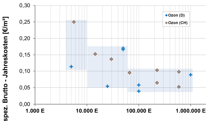
Bild 17: Spezifische Jahreskosten der Abwasser ozonung in Abhängigkeit der Ausbaugröße (ohne Berücksichtigung der Filter)
